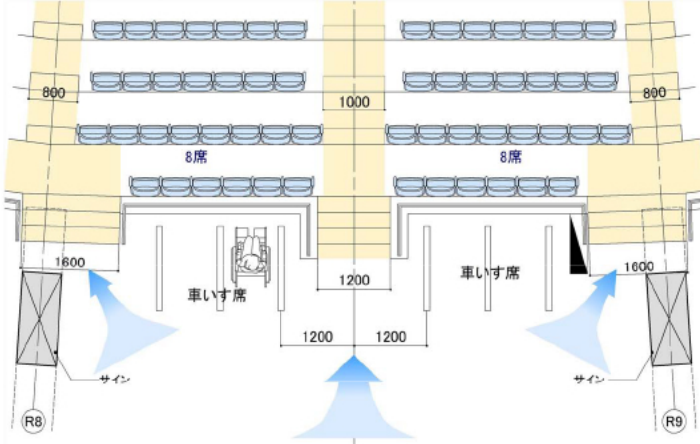
拡大図 (S=1/60)
