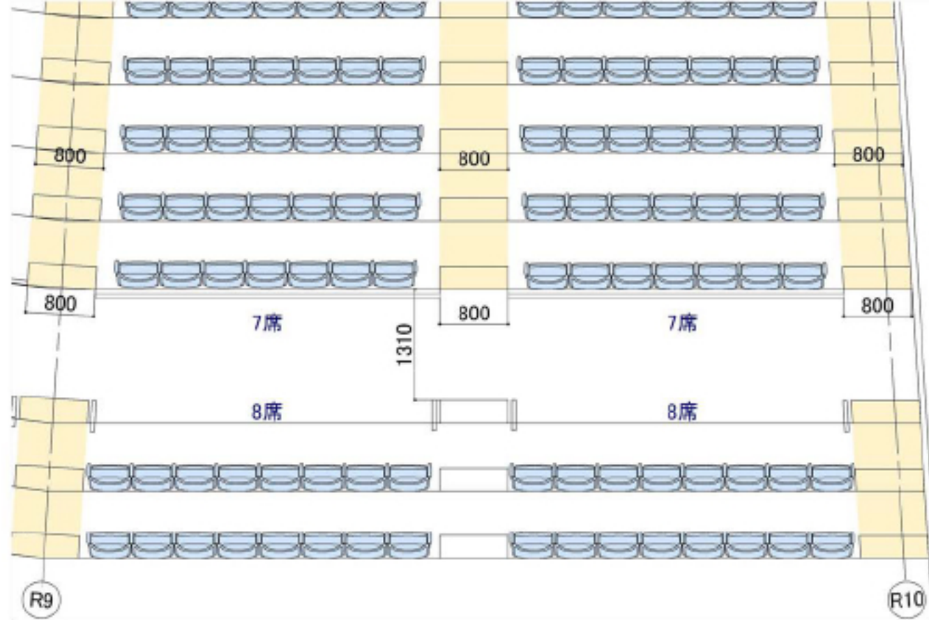
拡大図 (S=1/60)
